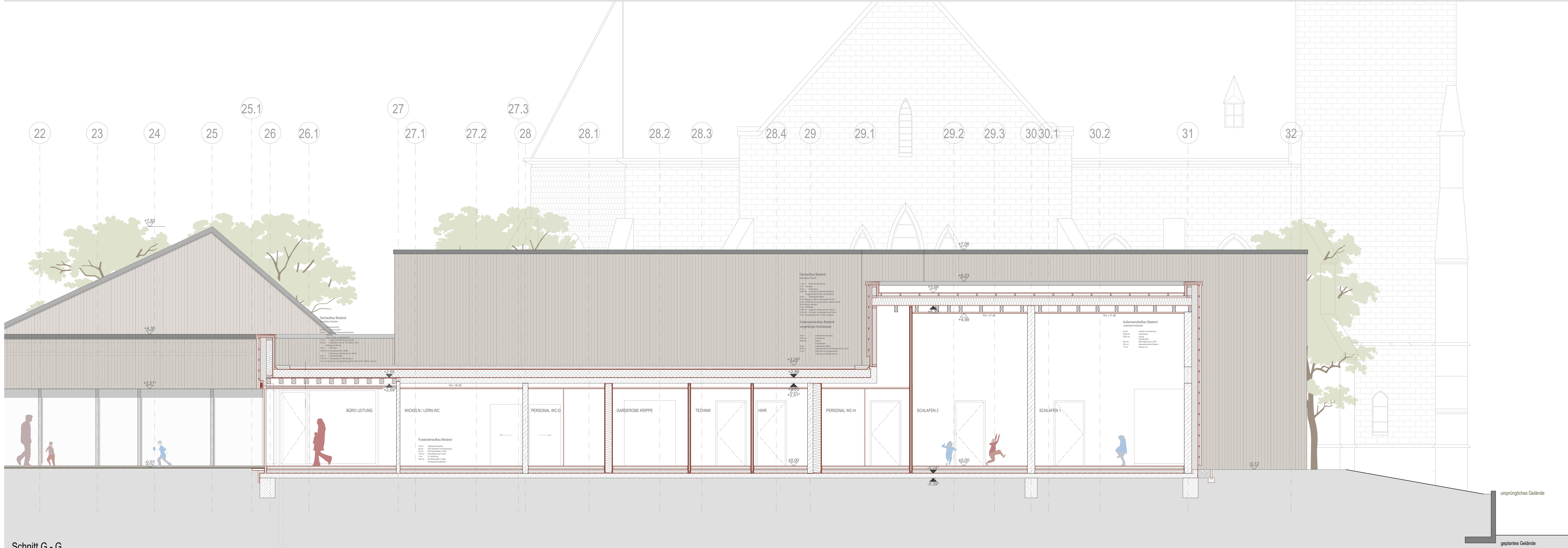
Schnitt G - G
